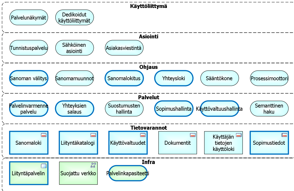
Integraatioratkaisun järjestelmäpino sekä kansallisen palveluväylän tarjoamat palvelut
